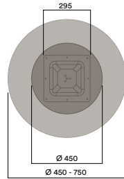
OTS-DB-1450-CT
