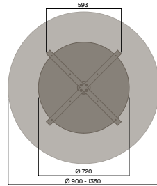
OTS-DB-1720
