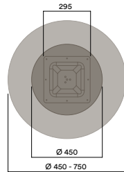
OTS-DB-1450
