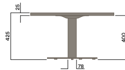
OTS-DB-1450
